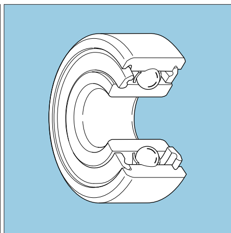
樹脂シール（非接触） SSA
